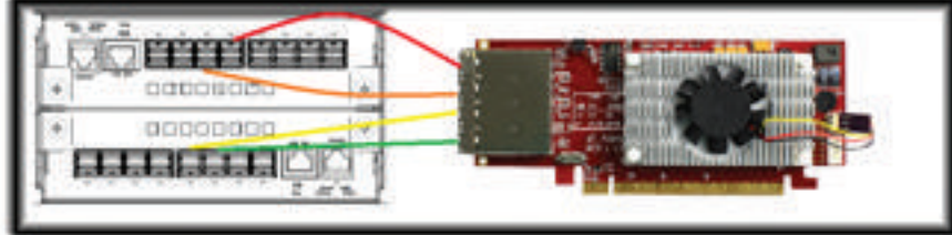
2x8 (Using SA-4444L Cables)
